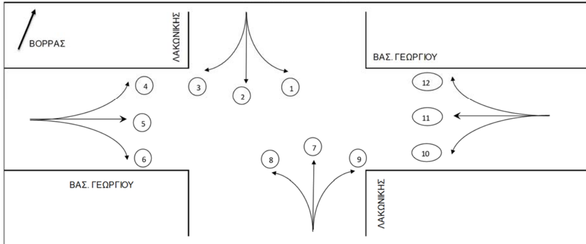
Σχεδιάγραμμα Διασταύρωσης
