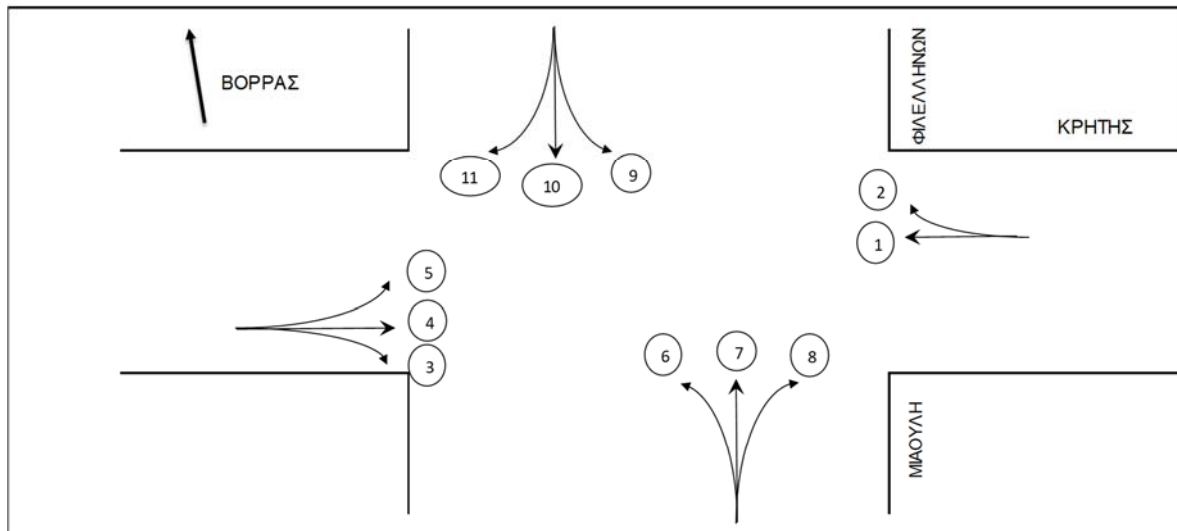
Σχεδιάγραμμα Διασταύρωσης
